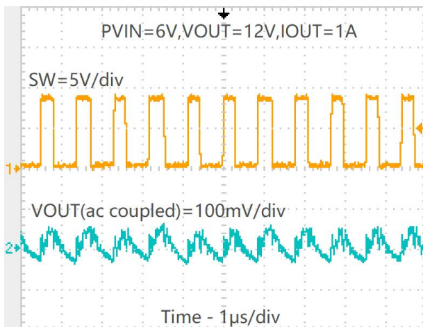
VOUT 纹波(PVIN=6V, VOUT=12V, IOUT=1A)
