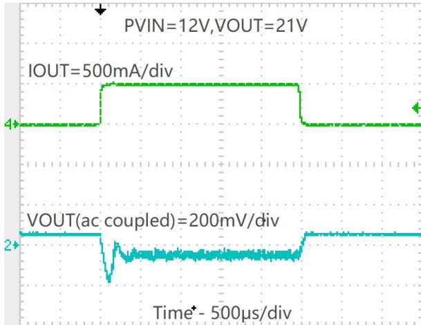
阶跃负载(PVIN=12V,VOUT=21V,IOUT=0 to 0.5A)
