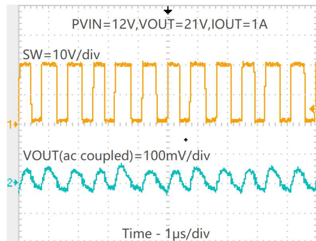
VOUT 纹波(PVIN=12V, VOUT=21V, IOUT=1A)
