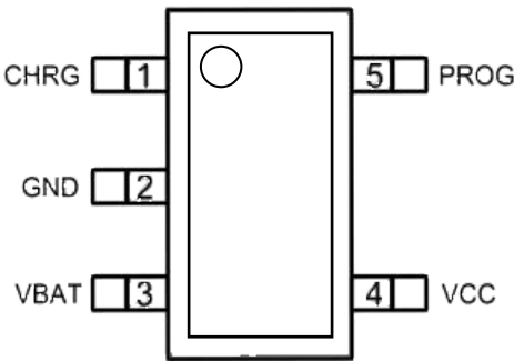
SOT23-5L
